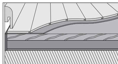
Ламинат на материале Uno-Protect / сухих деревянных полах
