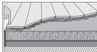
Полностью приклеенный ламинат Ламинат на материале Duo-Protect /
