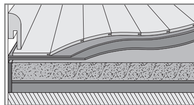
Ламинат на материале Uno-Protect / ПВХ или XВ / на минеральной стяжке
