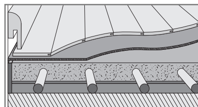
Обогрев пола горячей водой
