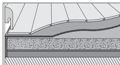
Ламинат на материале Duo-Protect / минеральной стяжке
